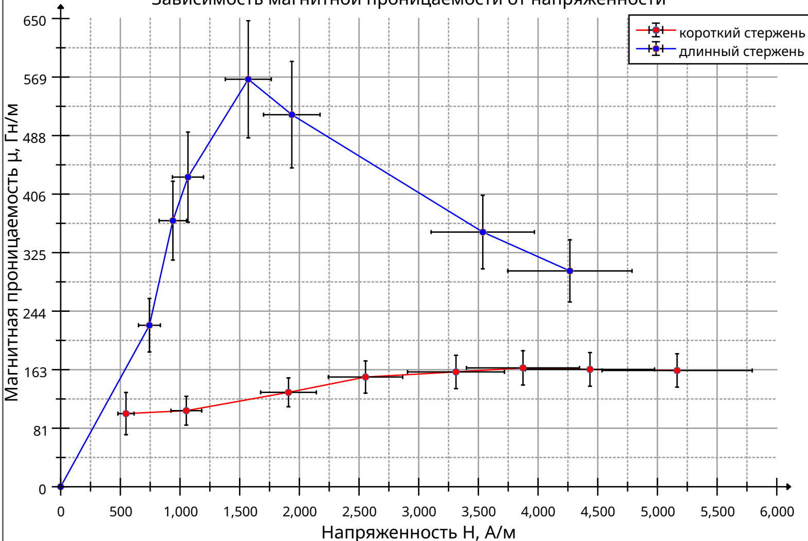
Зависимость магнитной проницаемости от напряженности
