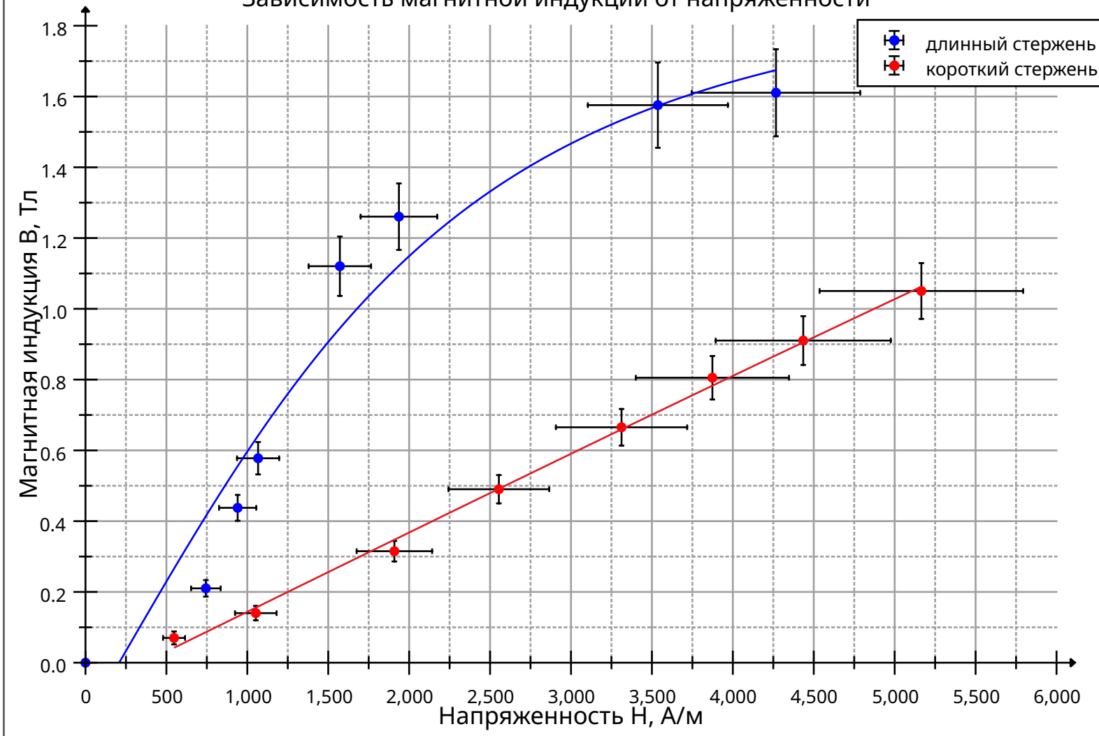
Зависимость магнитной индукции от напряженности
