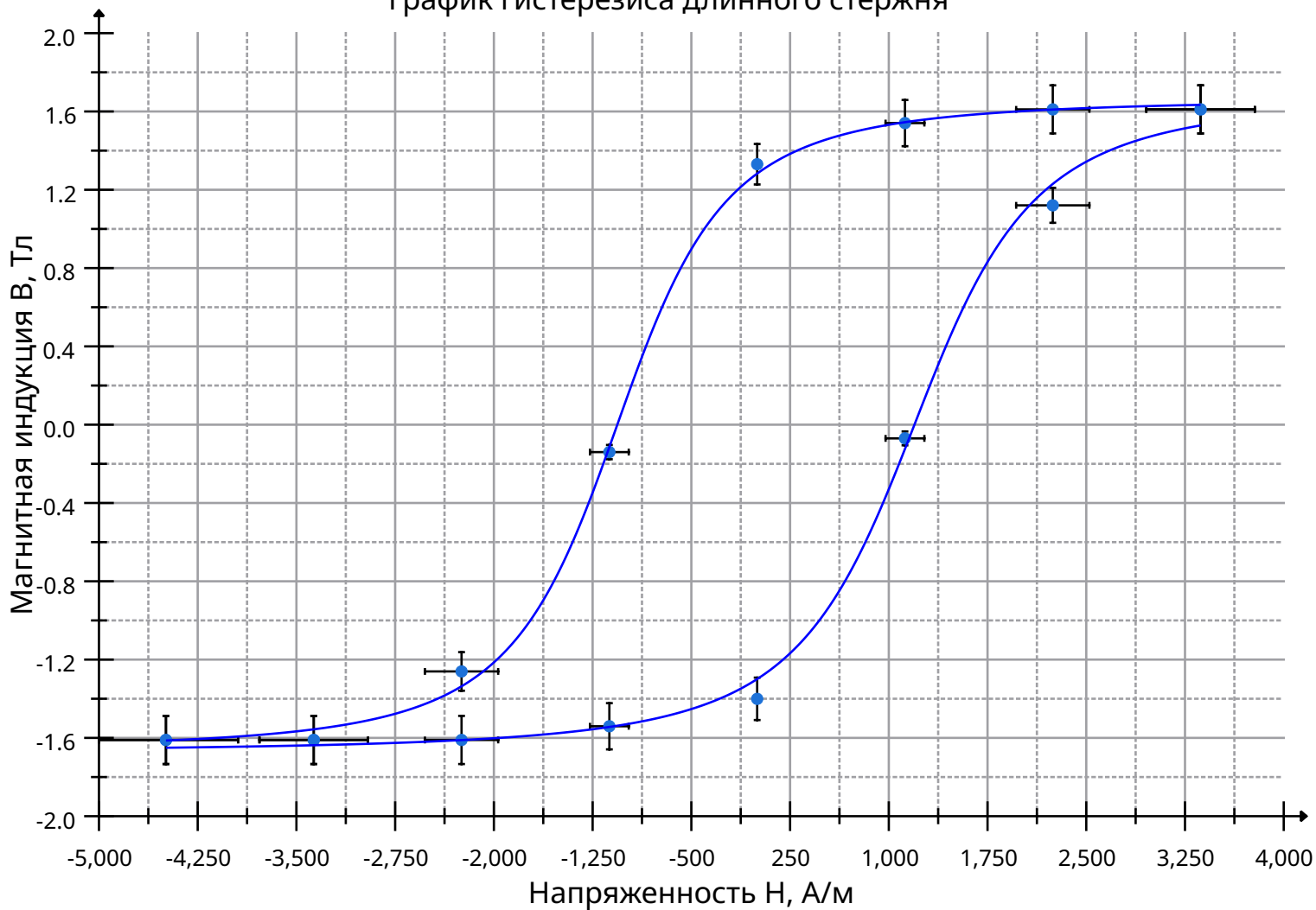
График гистерезиса длинного стержня
