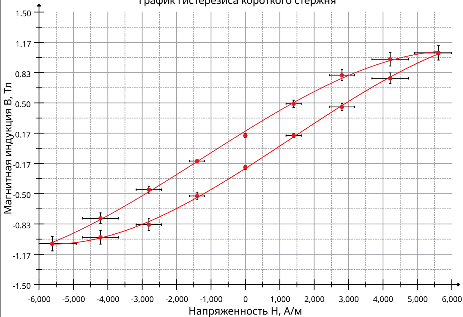
График гистерезиса короткого стержня
